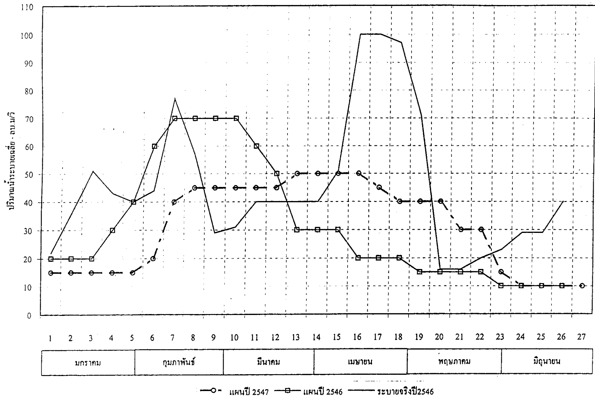
แผนการระบายจากอ่างเก็บน้ำเขื่อนป่าสักชลสิทธิ์ ในช่วงฤดูแล้ง ปี 2547
